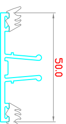
TRANSOM CAP 5000-SP16
